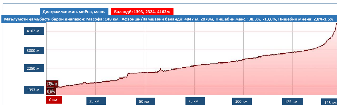
Расми 2.8. - Буриши тӯлии Фондарё
