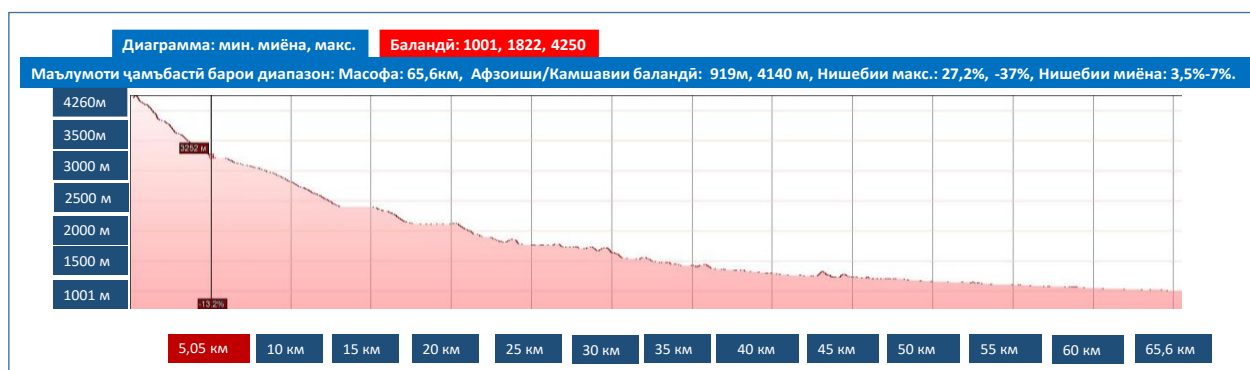
Расми 2.4. - Буриши тӯлии дарёи Шинг
