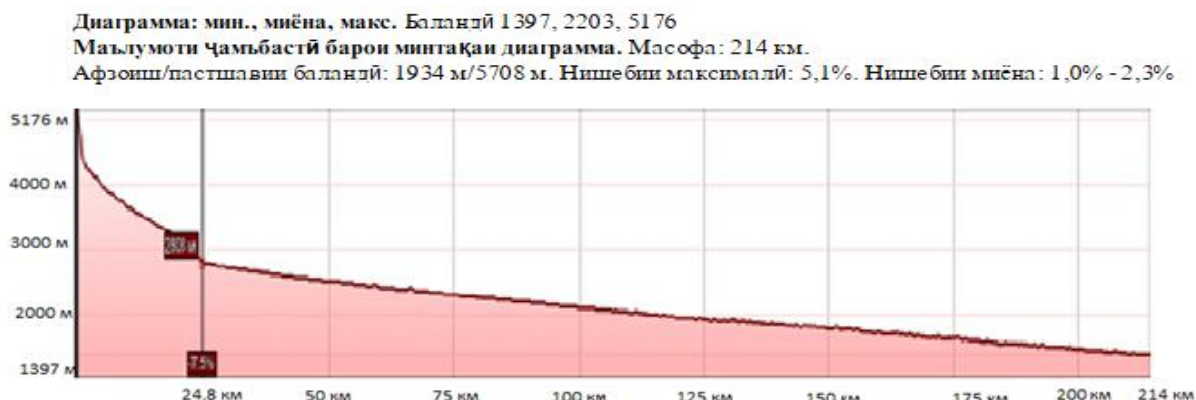
Расми 2.2. - Буриши тӯлии дарёи Масчоҳ (бо истифода аз барномаи Google Earth)
