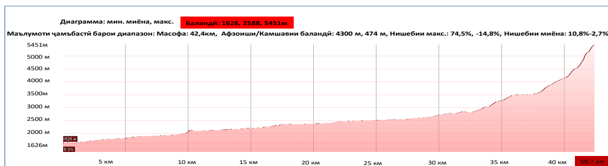
Расми 2.9. - Буриши тӯлии дарёи Пасруд
