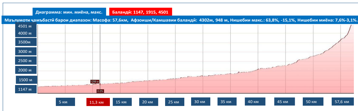
Расми 2.5. - Буриши тӯлии дарёи Киштуд
