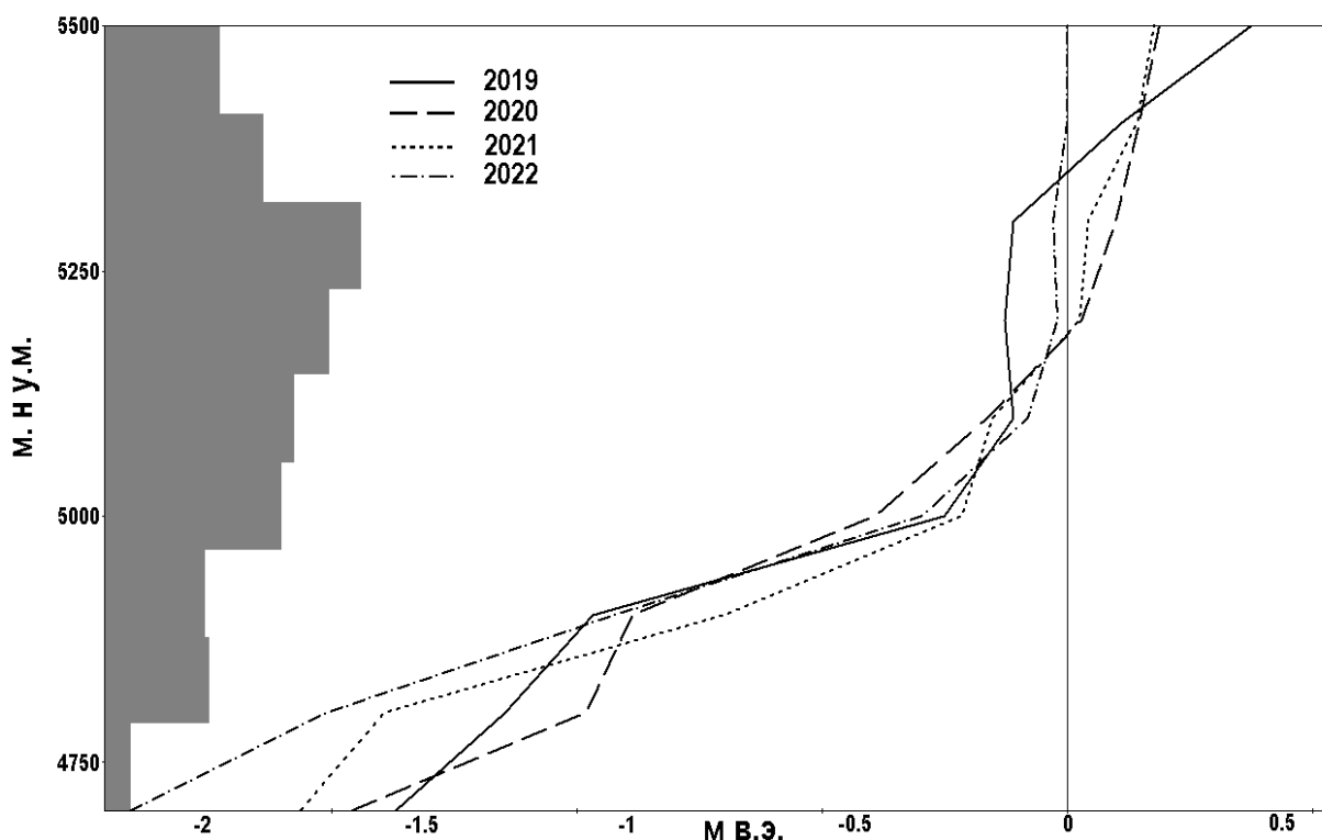
Рисунок 4.6. - Баланс массы профильным методом
