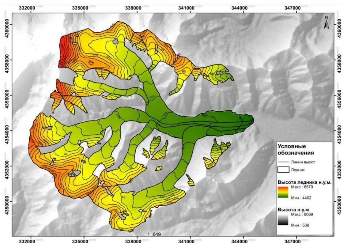
Рисунок 3.4. - Ледник Уйсу
