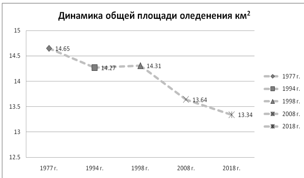
Рисунок 4.2. - Динамика площади оледенения.
