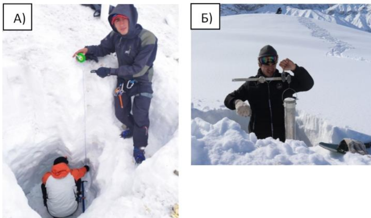
Рисунок 2.3. - Основные понятия полевых работ в зоне аккумуляции: А) Шурф в зоне аккумуляции; Б) Использование снегомера
