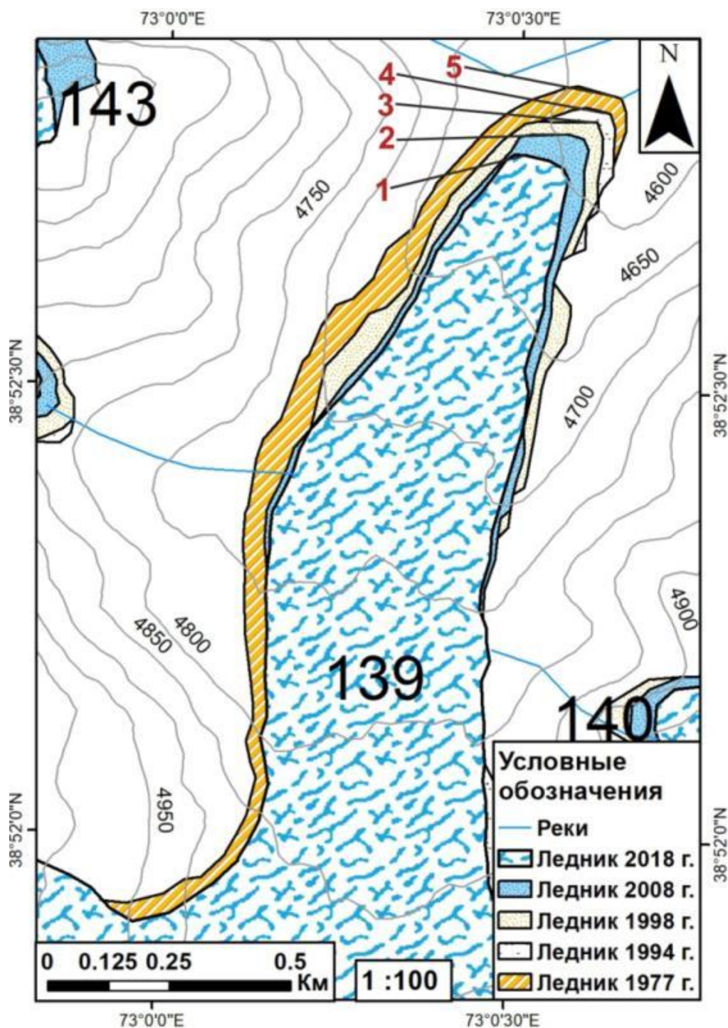
Рисунок 3.6. - Отступ ледника №139
