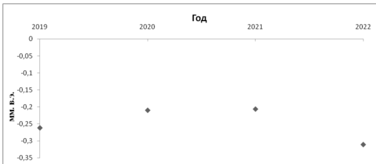
Рисунок 4.5. - Баланс массы методом изолиний
