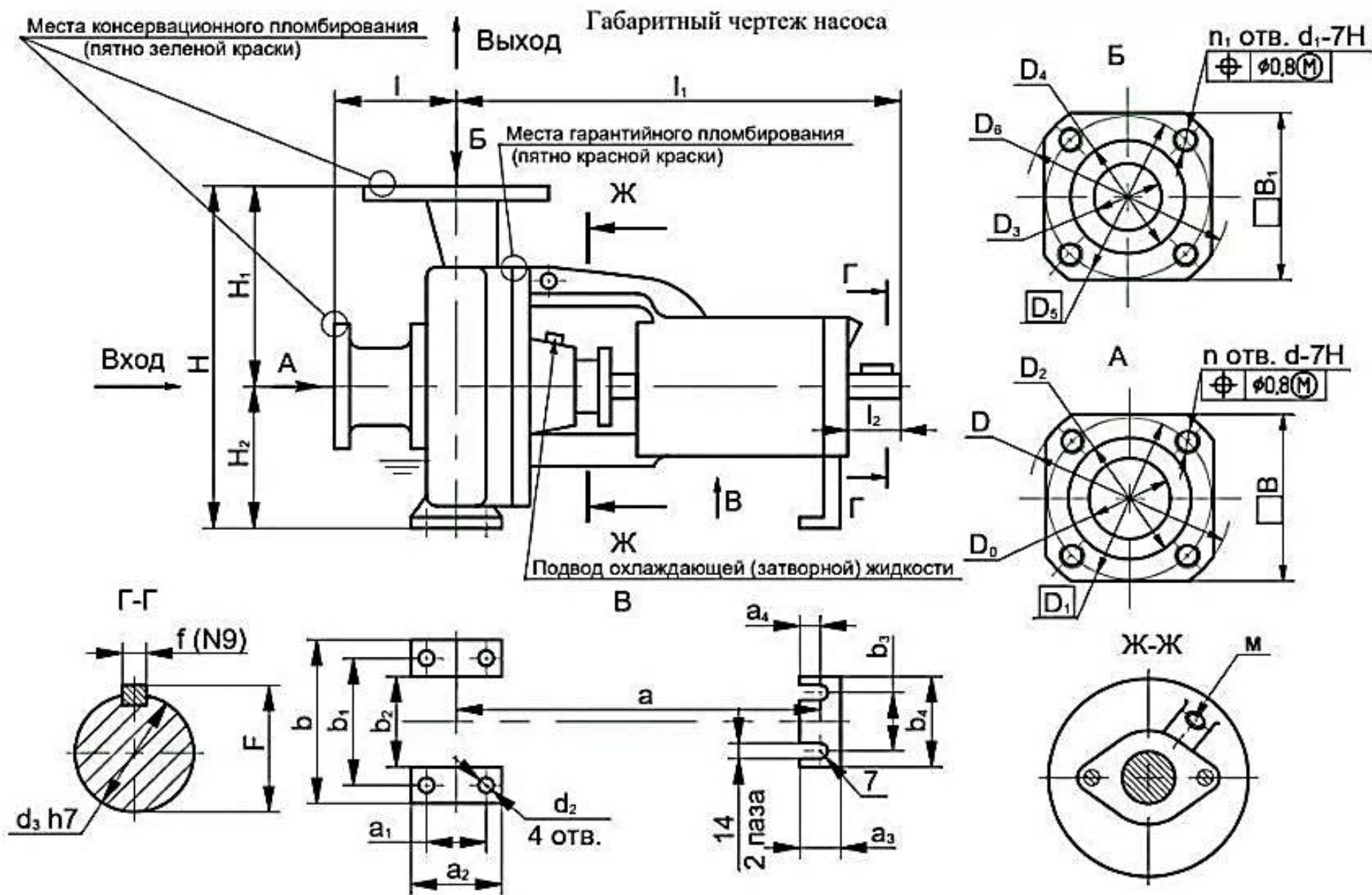
Рисунок 4.10. Габаритный чертеж насоса.
