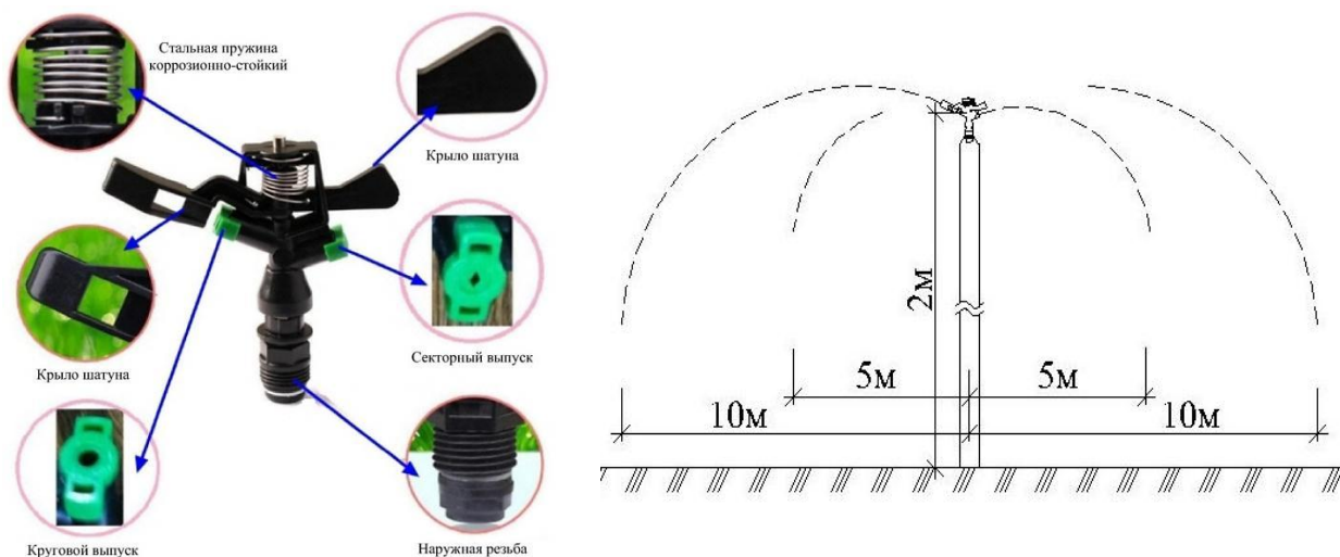
Рисунок 4.8. Схема усиленного дождевального аппарата на стоечных трубопроводах
