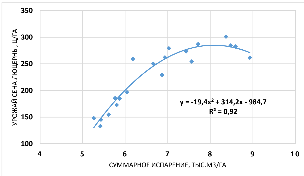
Рисунок 4.4. Зависимость урожая сена люцерны (Y, ц/га) от суммарного водопотребления (E, тыс. м³/га)
