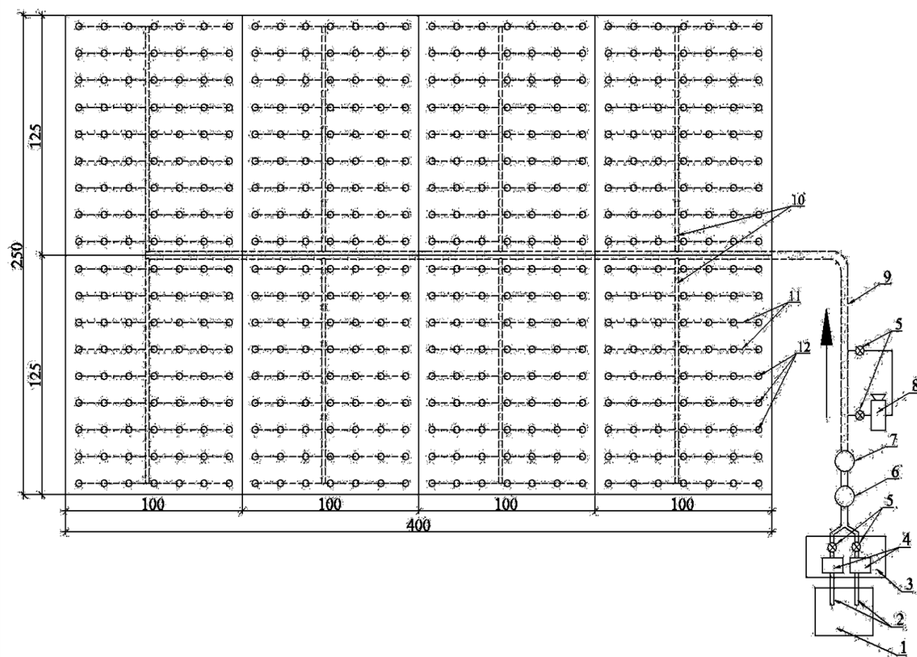
Рисунок 4.6. Принципиальная схема модульного участка стационарного дождевания люцерны
