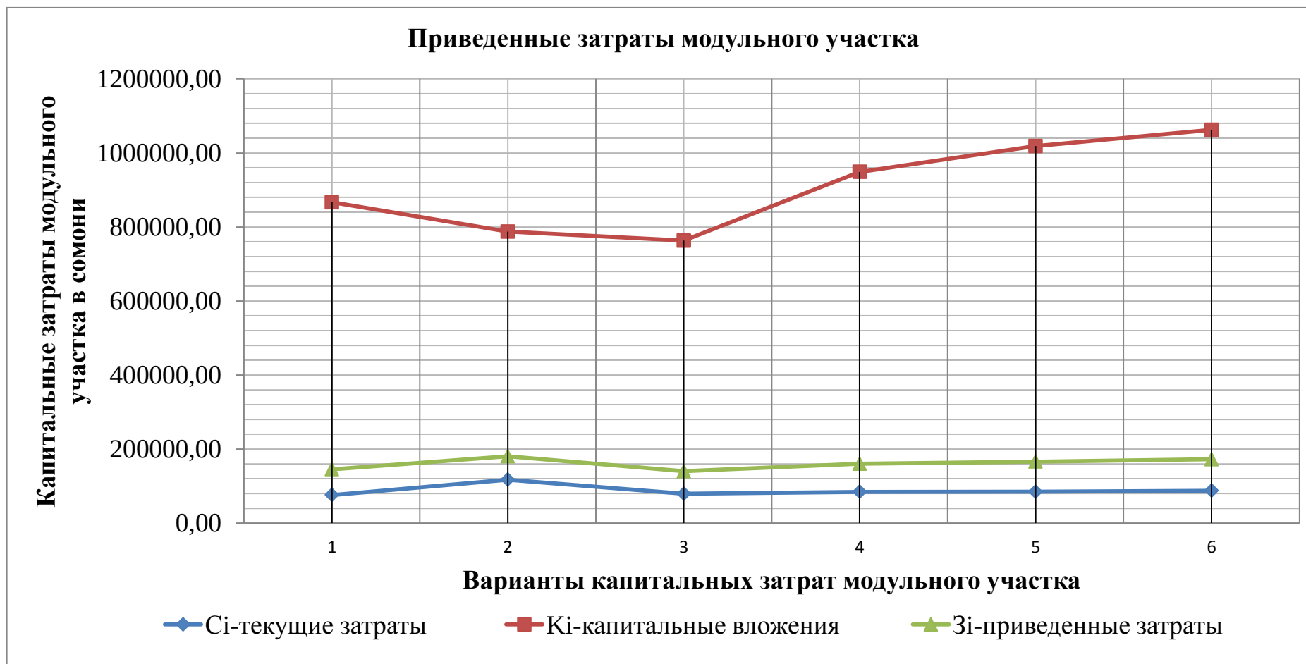
Рисунок 4.12. Приведенные затраты модульного участка
