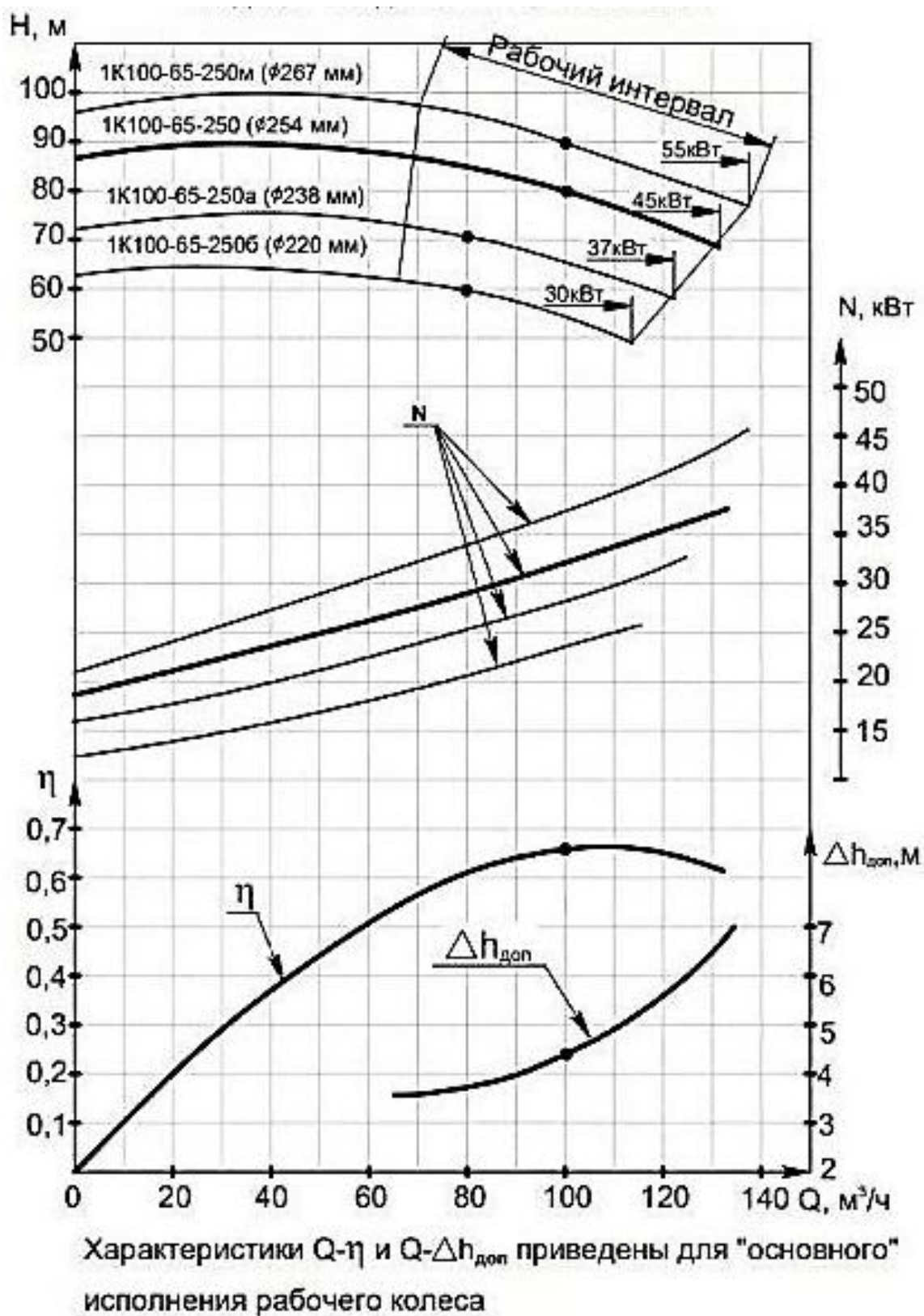
Рисунок 4.9. Рабочие характеристики насоса 1K100-65-250 при частоте вращения 2900 об./мин., жидкость – вода плотностью 1000 кг/м 3
