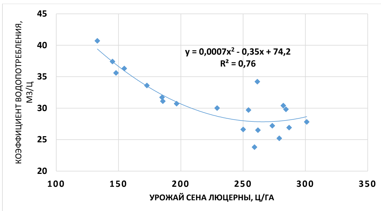
Рисунок 4.5. Зависимость коэффициента водопотребления (Kв, м³/ц) от урожая сена люцерны (Y, ц/га)
