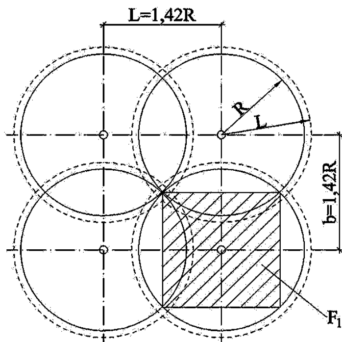
Рисунок 4.7. Принятая схема расположения дождевальных аппаратов
