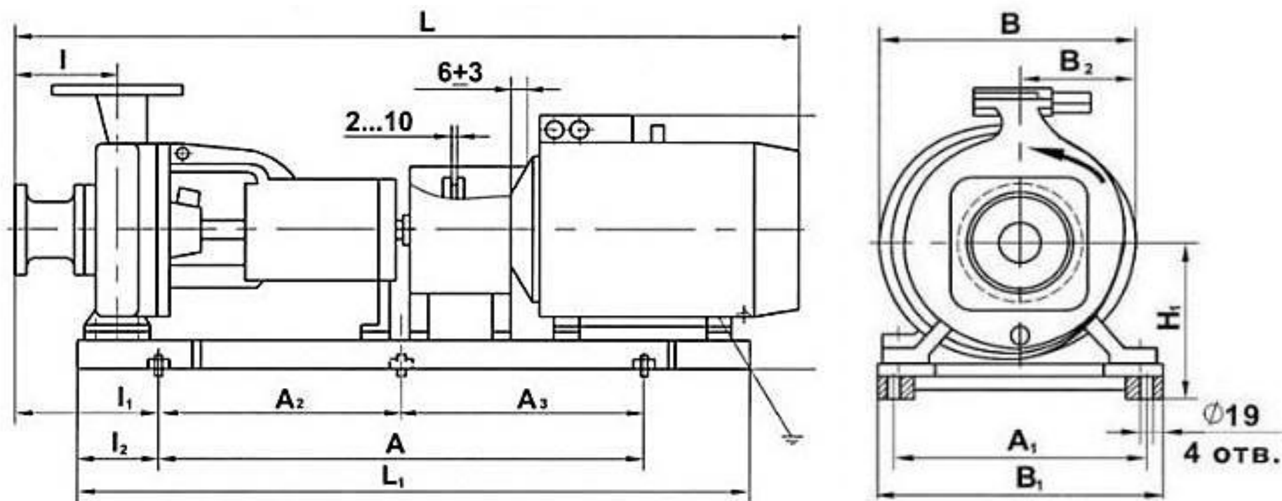
Рисунок 4.11. Габаритный чертеж насосного агрегата 1K100-65-250
