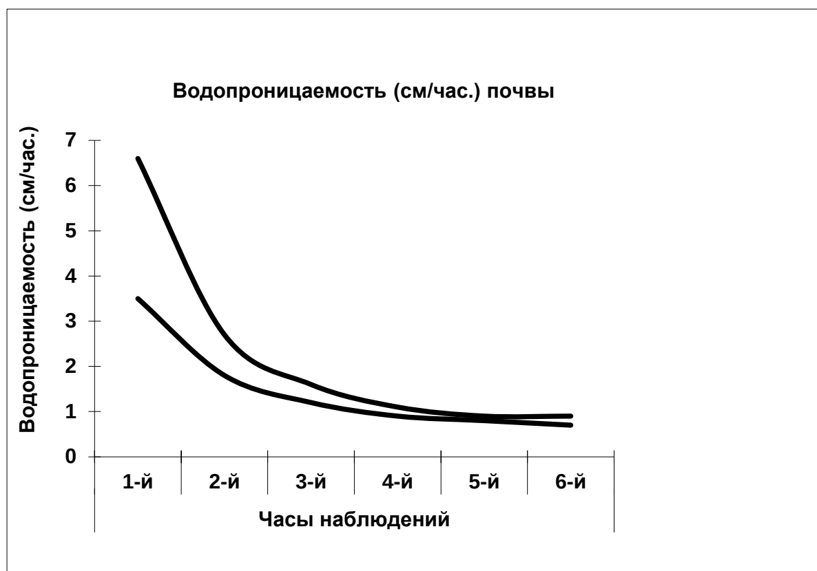
Рис.4.2. Водопрооницаемость среднесуглинистых и тяжелосуглинистых почв Центрального Таджикистана
